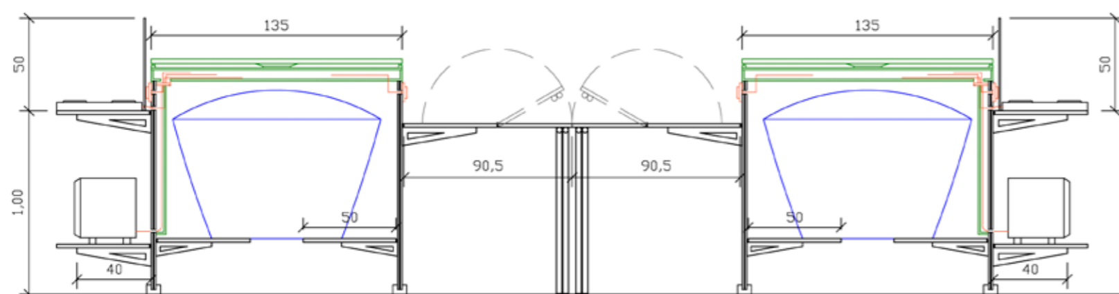
Corte equipamentos acoplados - Esc. 1:20
