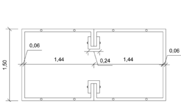
Detalhe da Peça central de Tração esc. 1:20 e 1:5
