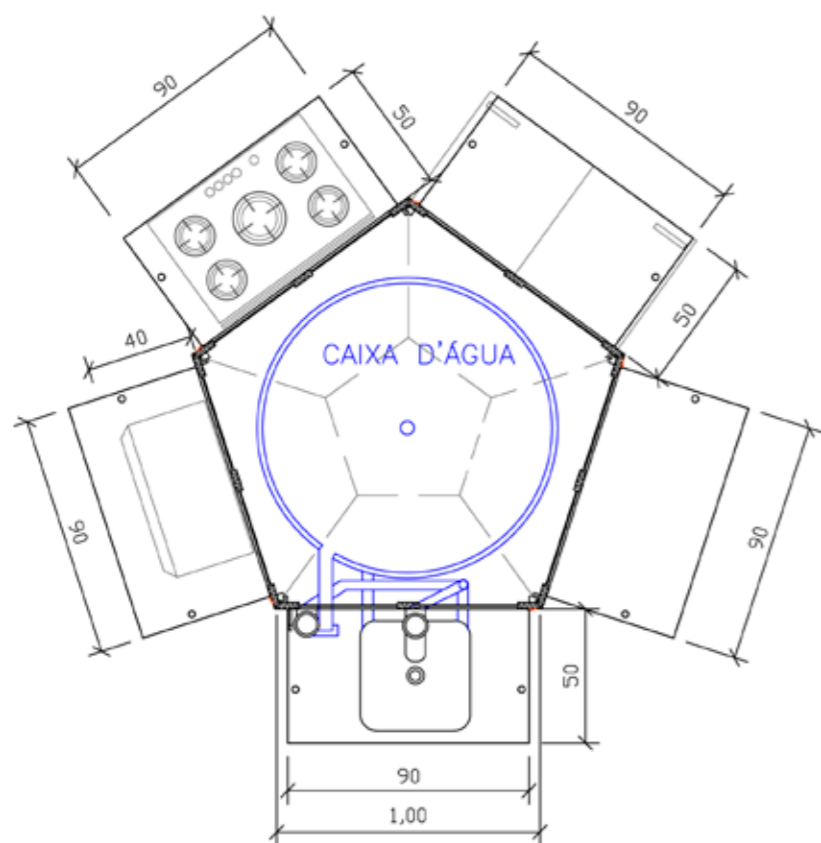
Planta equipamento - Cozinha - Esc. 1:20
