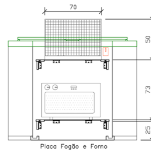
Modelo Eletrônico do módulo de cozinha
