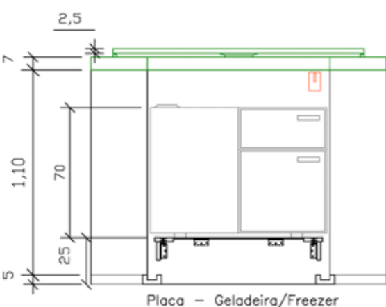
Vistas Frontais - Placas - Esc. 1:20
