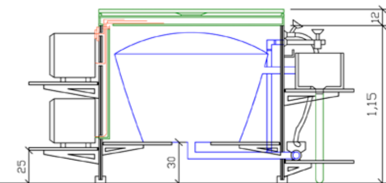
Corte equipamento simples - Esc. 1:20
