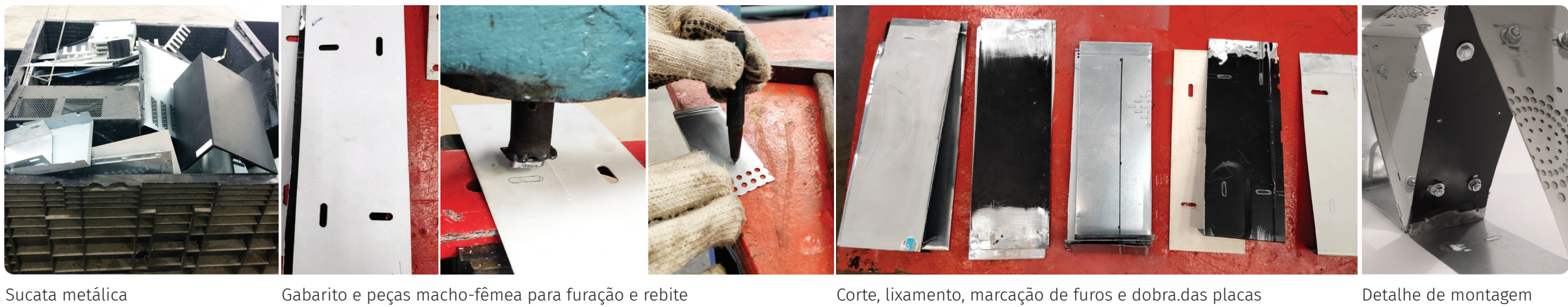
Sucata metálica
